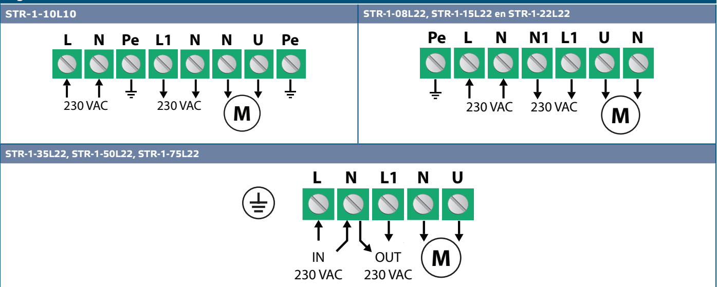
Fig.3 Aansluitschema
