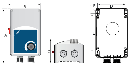
Fig. 1 Afmetingen
